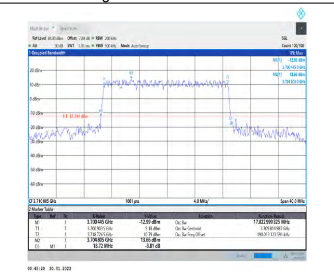
1-N78-3700-3800-30-20-L-4-DFT-64QAM-Outer_Full -50@0-Ant1-17.823-18.720-≤20-PASS
