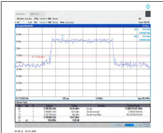
1-N78-3700-3800-30-20-L-3-DFT-16QAM-Outer_Full -50@0-Ant1-17.868-18.800-≤20-PASS
