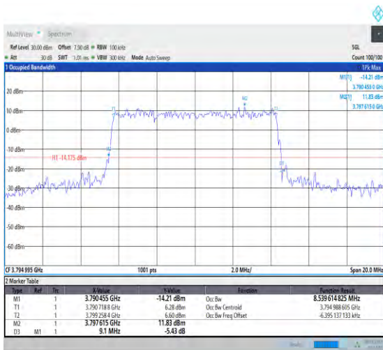
1-N78-3700-3800-30-10-H-3-DFT-16QAM-Outer_Ful I-24@0-Ant1-8.575-9.520-≤10-PASS
