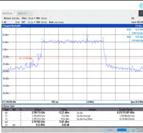
1-N78-3700-3800-30-10-H-3-DFT-16QAM-Outer_Ful I-24@0-Ant1-8.575-9.520-≤10-PASS
