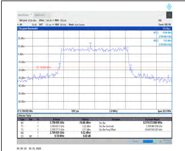
1-N78-3700-3800-30-10-L-9-CP-256QAM-Outer_Ful I-24@0-Ant1-8.574-9.180-≤10-PASS
