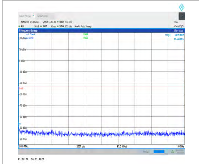
1-N66-PC3-15-40-H-1-DFT-PI2BPSK-Inner_1RB_L eft-1@1-30-1000-Ant1-31.46--59.99--23-PASS
