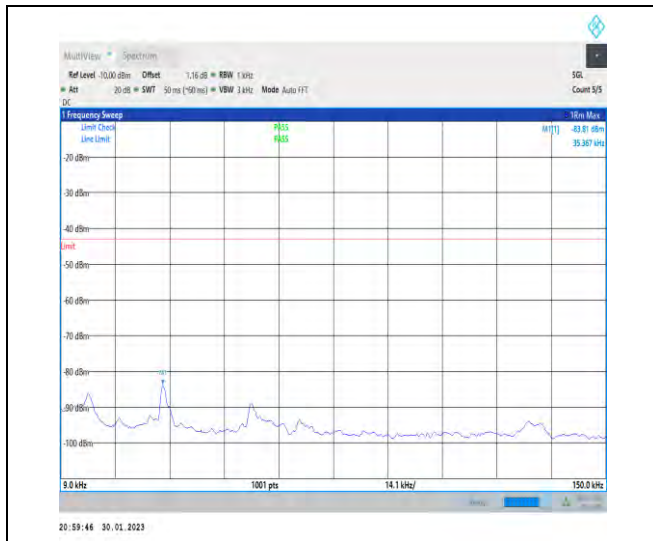
1-N66-PC3-15-40-H-1-DFT-PI2BPSK-Inner_1RB_L eft-1@1-0.009-0.15-Ant1-0.04--83.81--43-PASS
