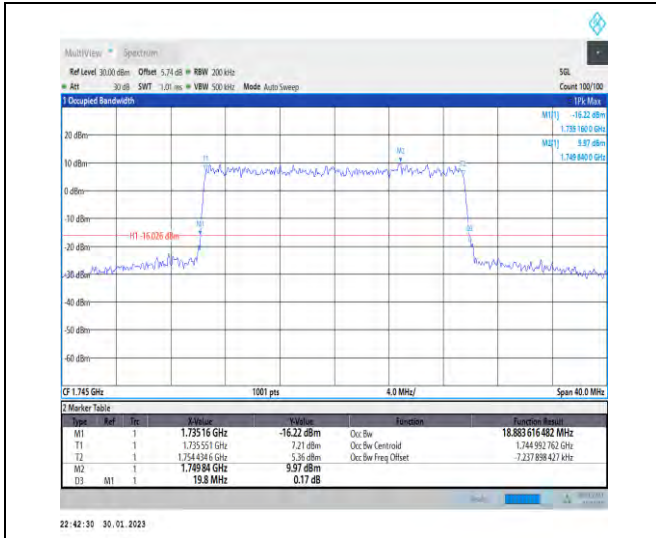
1-N66-PC3-15-20-M-7-CP-16QAM-Outer_Full-106@ 0-Ant1-18.884-19.800-≤20-PASS
