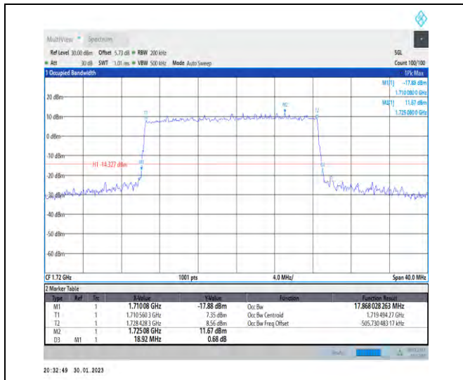
1-N66-PC3-15-20-L-4-DFT-64QAM-Outer_Full-100 @0-Ant1-17.868-18.920-≤20-PASS
