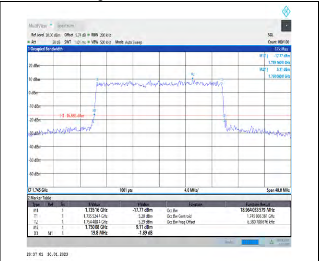
1-N66-PC3-15-20-M-8-CP-64QAM-Outer_Full-106@ 0-Ant1-18.964-19.800-≤20-PASS
