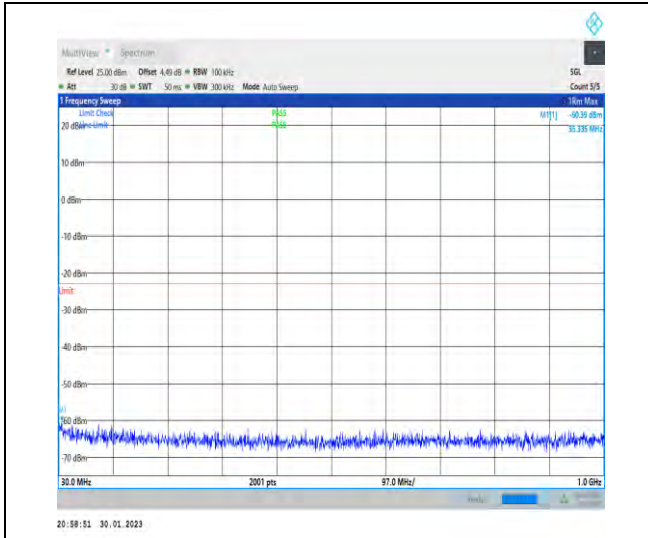
1-N66-PC3-15-40-M-1-DFT-PI2BPSK-Inner_1RB_L eft-1@1-30-1000-Ant1-35.34--60.39--23-PASS
