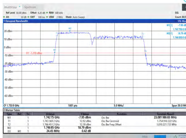
66-66-10MHz-15MHz-QPSK-QPSK-132351-132471-50RB#0-75RB#0
