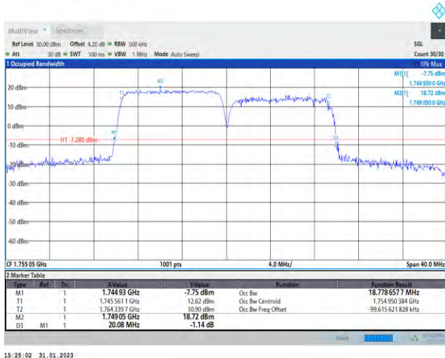
66-66-10MHz-10MHz-QPSK-QPSK-132373-132472-50RB#0-50RB#0
