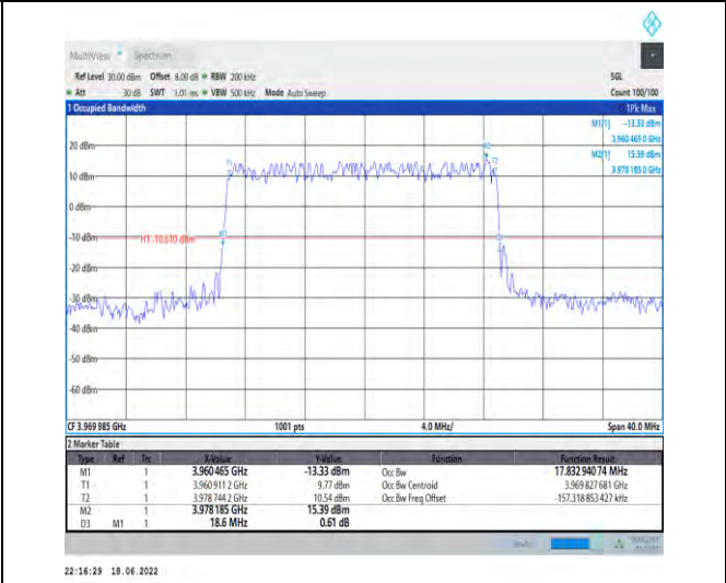
1-N77-3700-3980--30-20-H-2-DFT-PI2BPSK-Outer_Full -50@0-Ant1-17.833-18.600-<20-PASS
