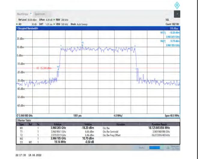
1-N77-3700-3980--30-20-H-6-CP-QPSK-Outer_Full-50@0-Ant1-18.126-19.160-≤20-PASS
