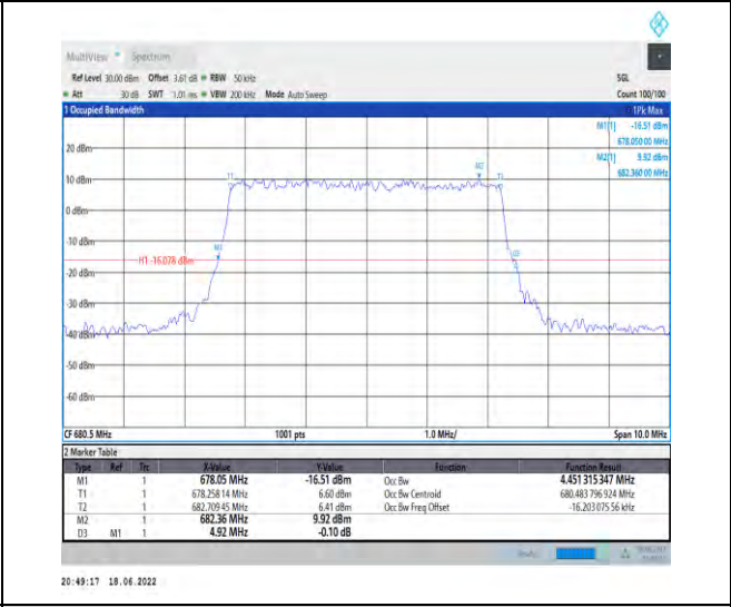
1-N71--15-5-M-7-CP-16QAM-Outer_Full-25@0-Ant1 -4.451-4.920-≤5-PASS
