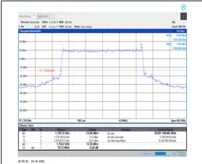
1-N66--15-20-M-7-CP-16QAM-Outer_Full-106@0-A nt1-18.931-19.720-≤20-PASS
