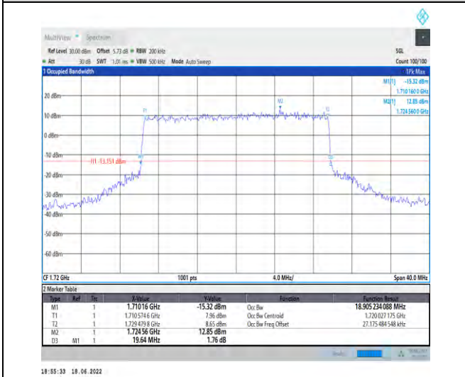
1-N66--15-20-L-6-CP-QPSK-Outer_Full-106@0-Ant1 -18.905-19.640-≤20-PASS
