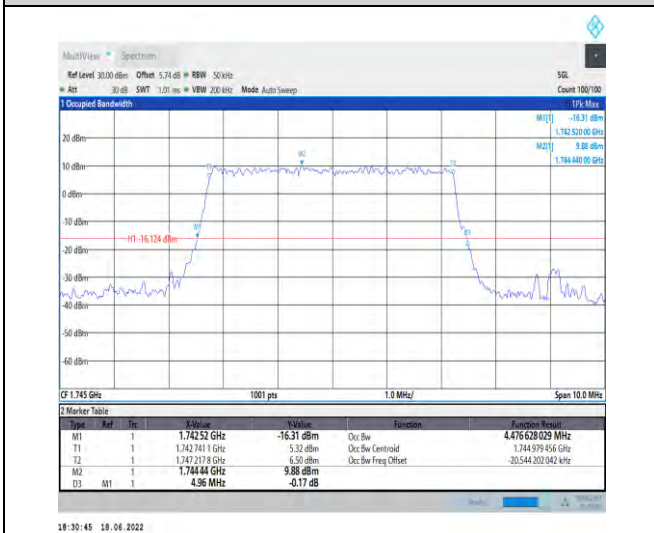
1-N66--15-5-M-6-CP-QPSK-Outer_Full-25@0-Ant1 4.477-4.960-≤5-PASS
