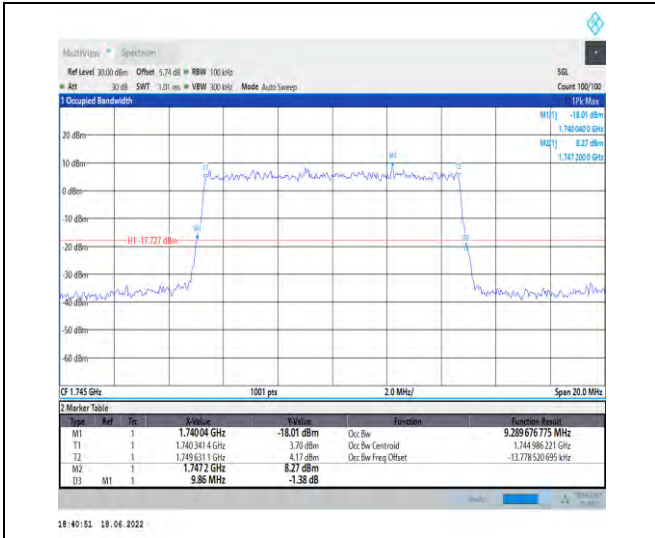
1-N66--15-10-M-9-CP-256QAM-Outer_Full-52@0-A nt1-9.29-9.860-≤10-PASS
