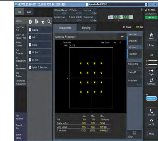
1-N66-PC3-15-40-M-7-CP-16QAM-Outer_Full-216@ 0-Ant1-see graph-PASS
