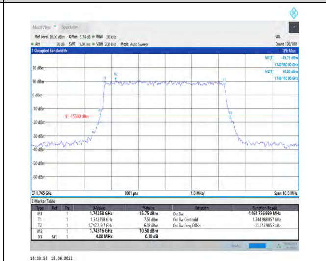
1-N66--15-5-M-7-CP-16QAM-Outer_Full-25@0-Ant1 -4.462-4.880-≤5-PASS
