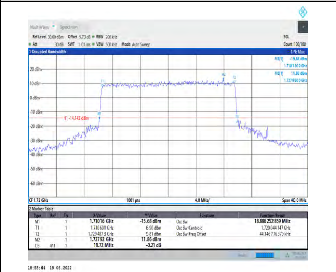
1-N66--15-20-L-7-CP-16QAM-Outer_Full-106@0-Ant1 t1-18.886-19.720-≤20-PASS
