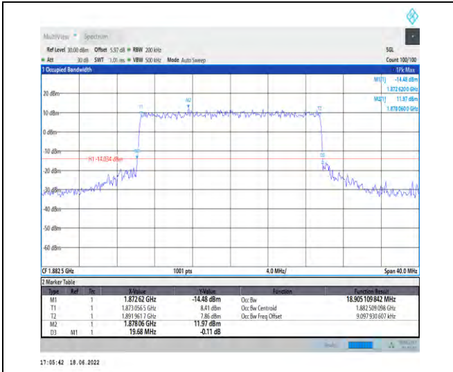
1-N25-PC3-15-20-M-7-CP-16QAM-Outer_Full-106@ 0-Ant1-18.905-19.680-≤20-PASS
