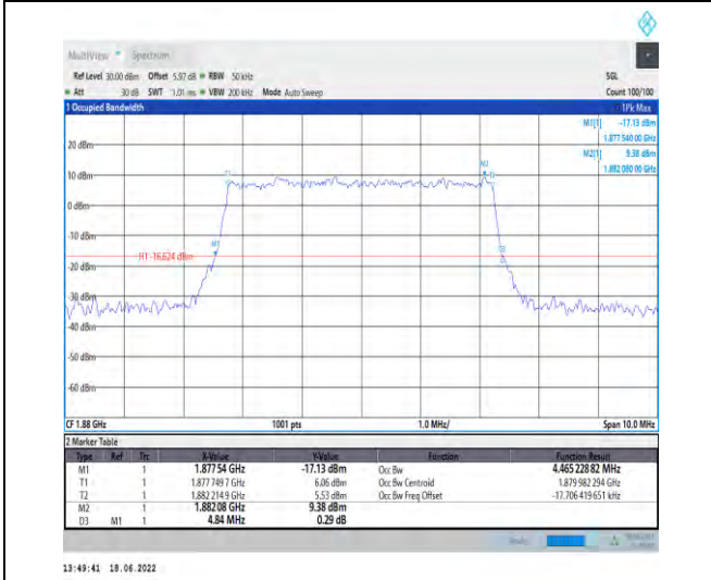
1-N2--15-5-M-6-CP-QPSK-Outer_Full-25@0-Ant1-4. 465-4.840-≤5-PASS
