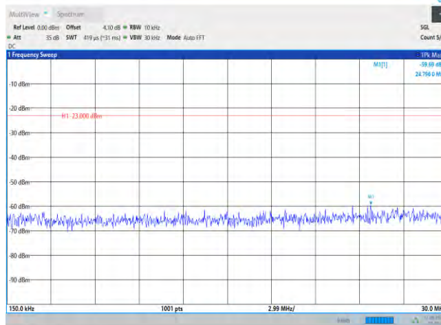
Band66-20MHz-QPSK-132072-1RB#0-Range2:0.15~30MHz
