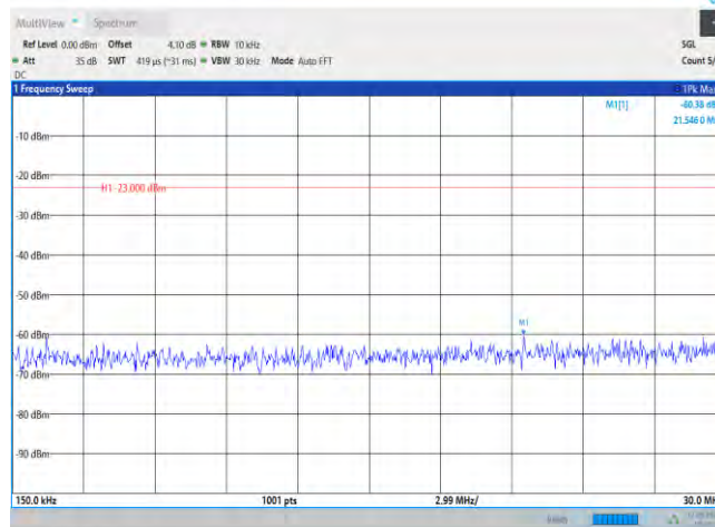
Band25-20MHz-QPSK-26140-1RB#0-Range2:0.15~30MHz
