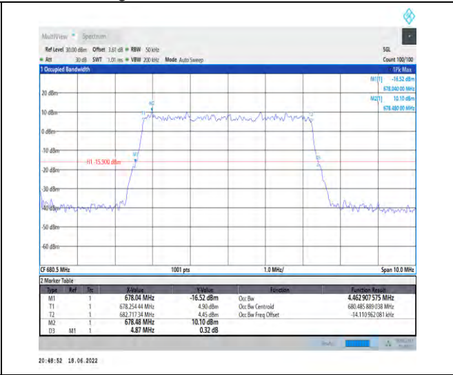
1-N71--15-5-M-5-DFT-256QAM-Outer_Full-25@0-A nt1-4.463-4.870-≤5-PASS
