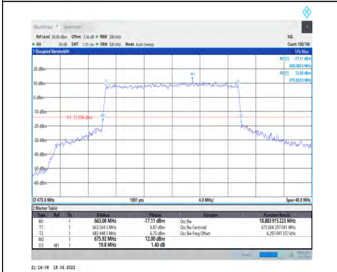
1-N71--15-20-L-6-CP-QPSK-Outer_Full-106@0-Ant1 -18.884-19.800-≤20-PASS
