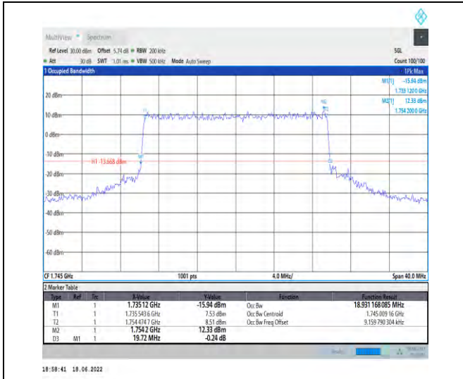
1-N66--15-20-M-7-CP-16QAM-Outer_Full-106@0-A nt1-18.931-19.720-≤20-PASS
