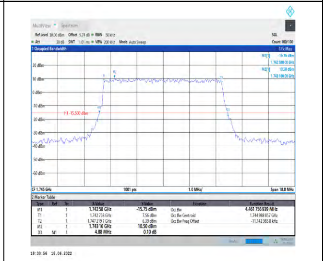
1-N66--15-5-M-7-CP-16QAM-Outer_Full-25@0-Ant1 -4.462-4.880-≤5-PASS
