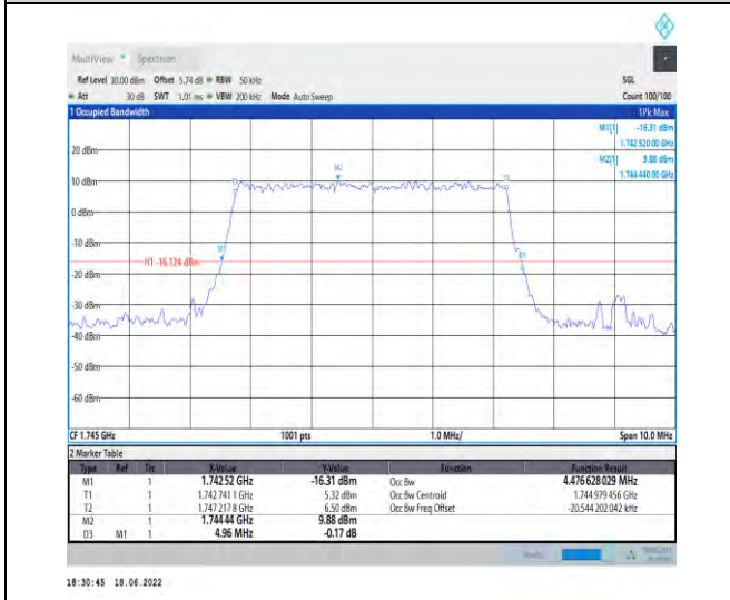
1-N66--15-5-M-6-CP-QPSK-Outer_Full-25@0-Ant1 4.477-4.960-≤5-PASS
