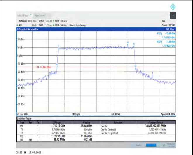
1-N66--15-20-L-7-CP-16QAM-Outer_Full-106@0-Ant1 t1-18.886-19.720-≤20-PASS
