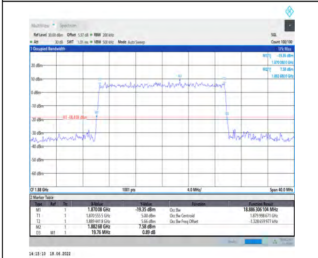
1-N2--15-20-M-9-CP-256QAM-Outer_Full-106@0-A nt1-18.886-19.760-≤20-PASS
