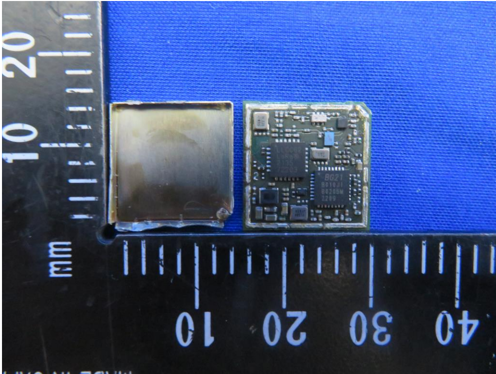
(5) EUT Photo(KG100SAAMD)
