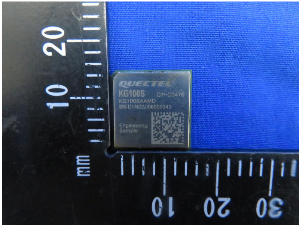
(3) EUT Photo(KG100SAAMD)
