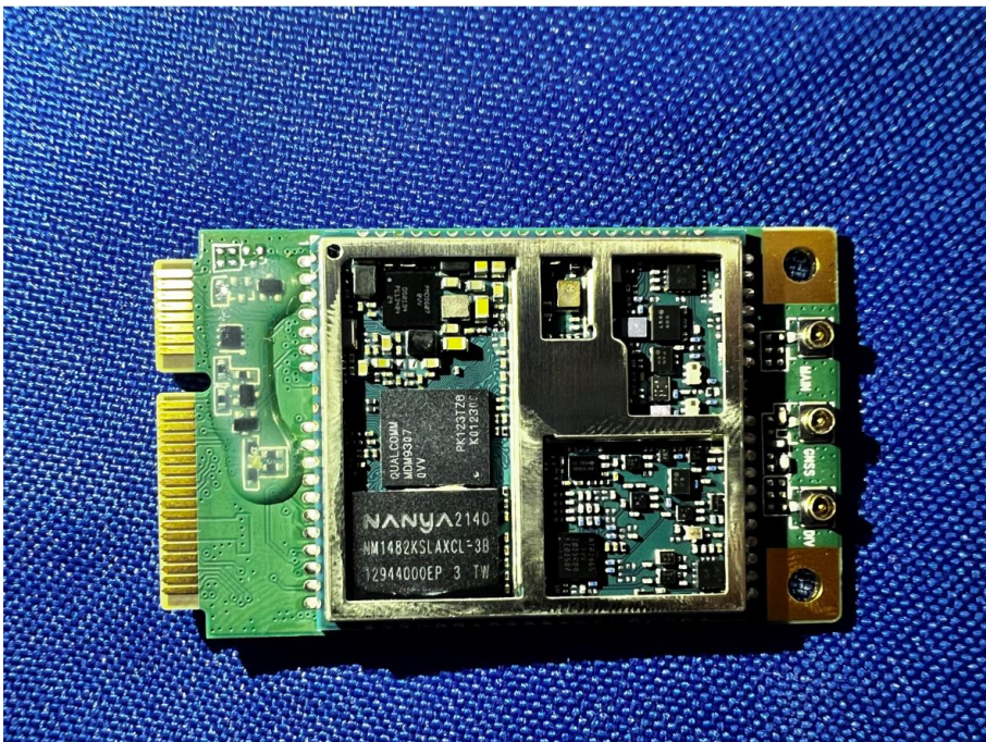
(4) EUT Photo (EC25-AFDL MINIPCI-E)
