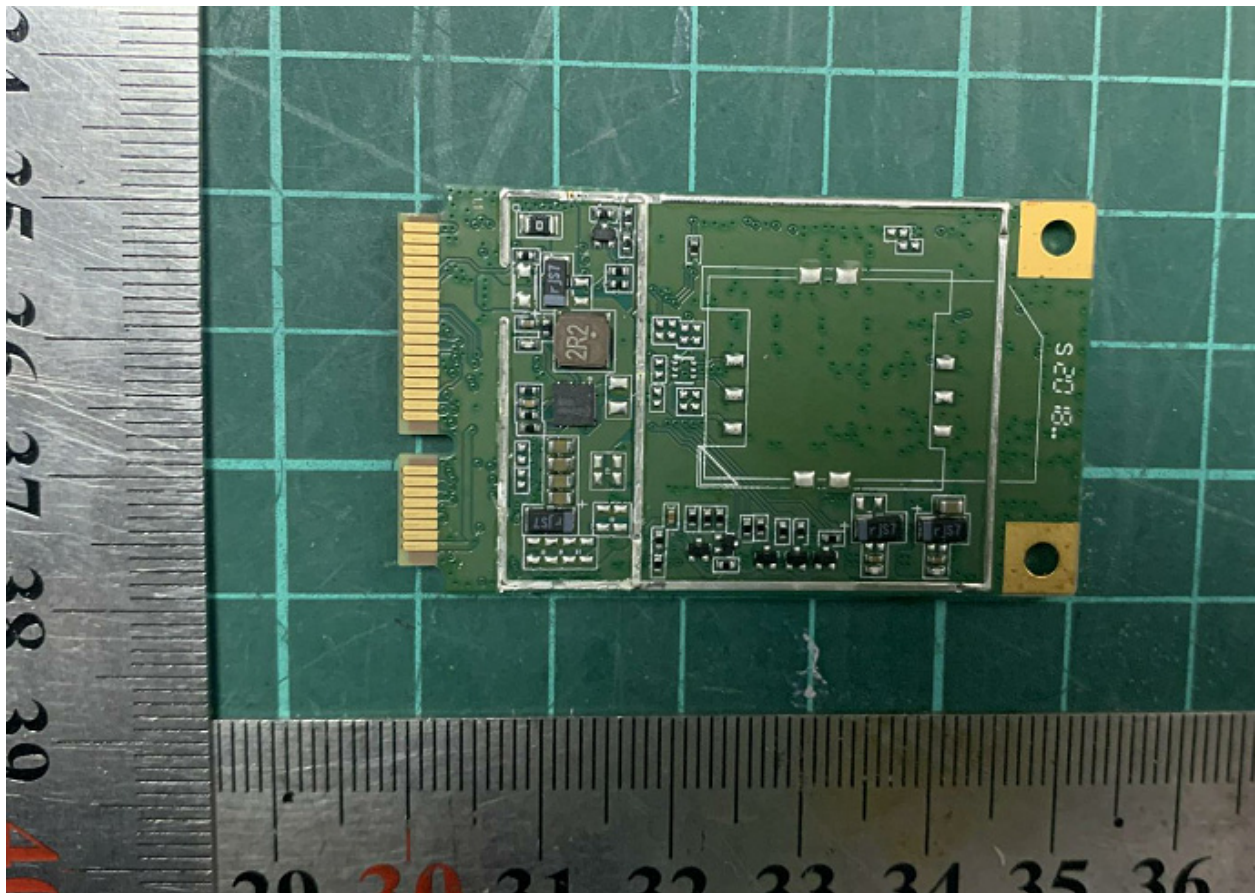
EC200T-AU MINIPCIE
