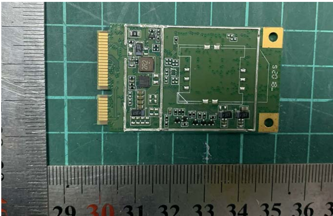
EC200T-AU MINIPCIE
