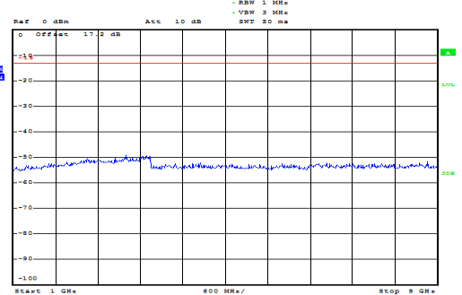
WCDMA Band V CH-Low 1GHz ~ 9GHz
