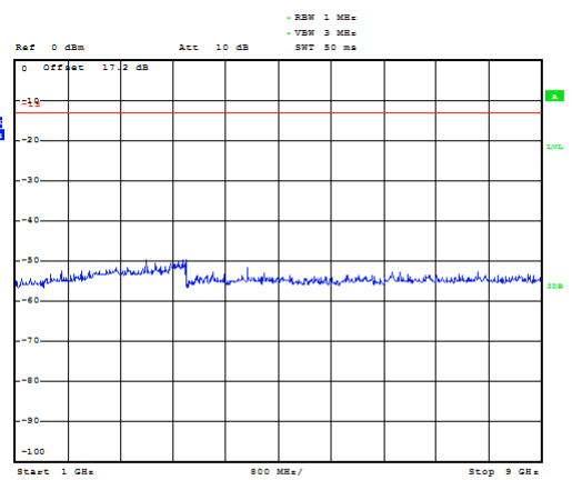
WCDMA Band V CH-High 1GHz ~ 9GHz
