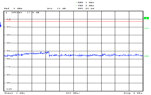
WCDMA Band V CH-Middle 1GHz ~ 9GHz
