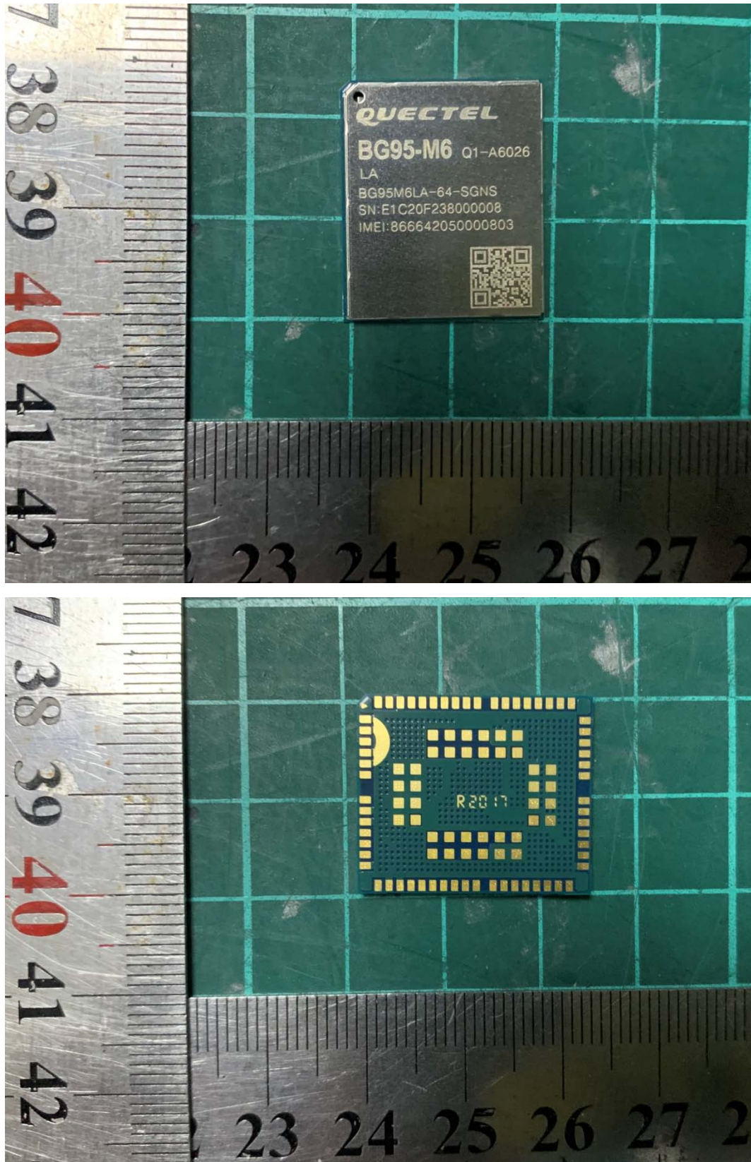
a: EUT
