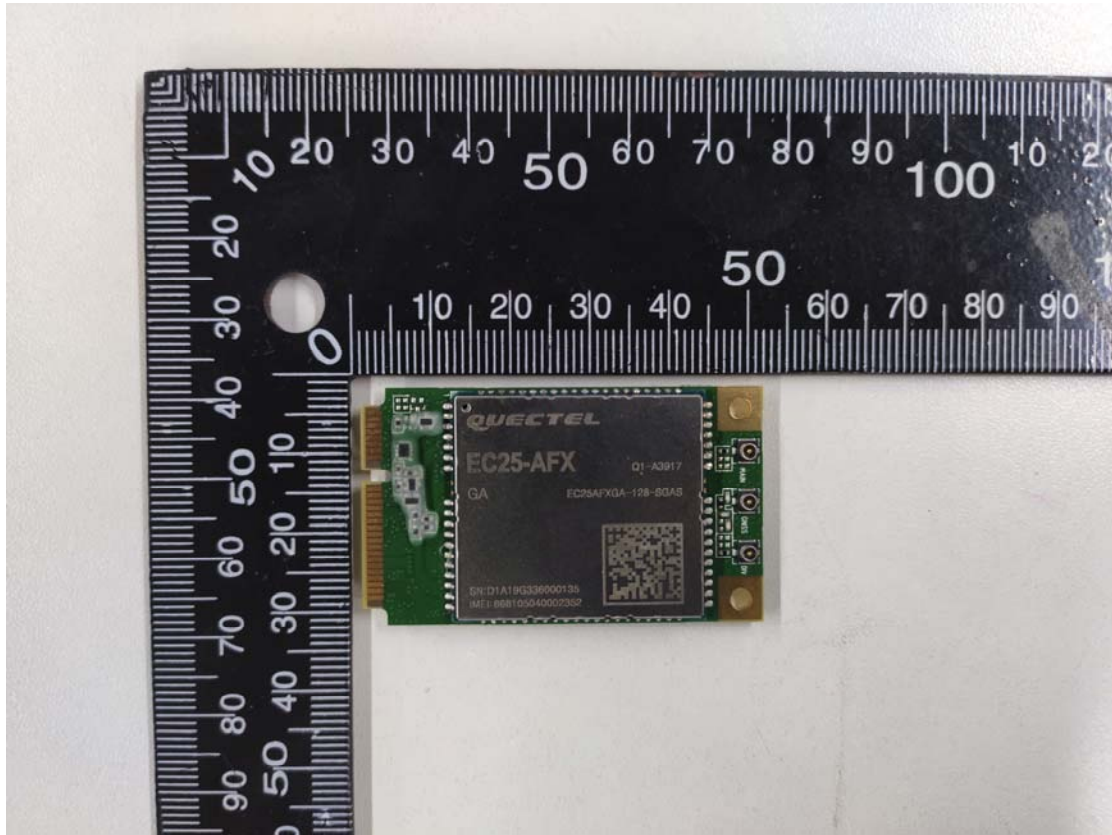
EC25-AFX MINIPCIE
