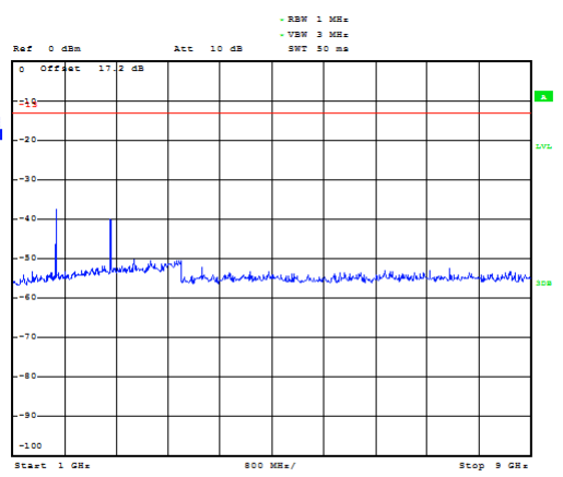
WCDMA Band V CH-Middle 1GHz ~ 9GHz
