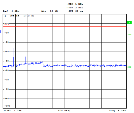
WCDMA Band V CH-Low 1GHz ~ 9GHz
