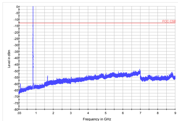
WCDMA Band V CH-Middle 30MHz ~ 9GHz
