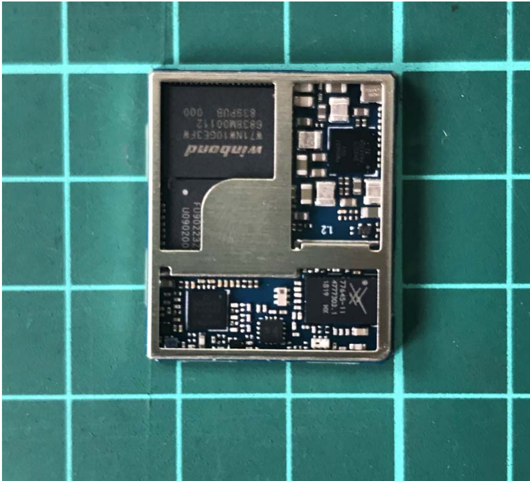
a: EUT
