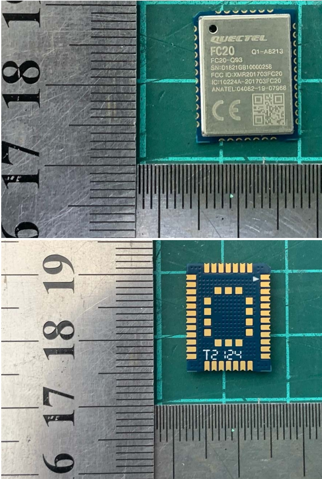
a: EUT
