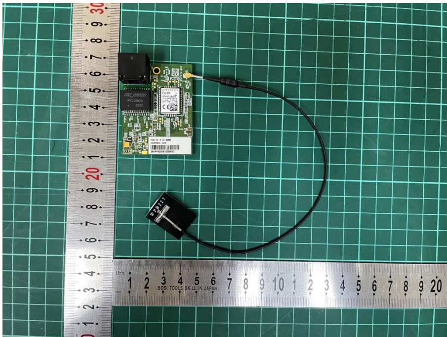
Antenna 3(45-2-000368)
