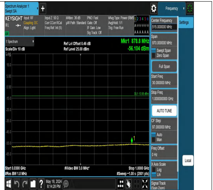
Band4-1413-2-30~1000MHz-PASS
