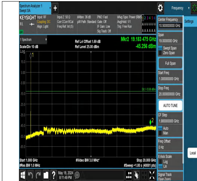
Band4-1312-1-1000~20000MHz-PASS
