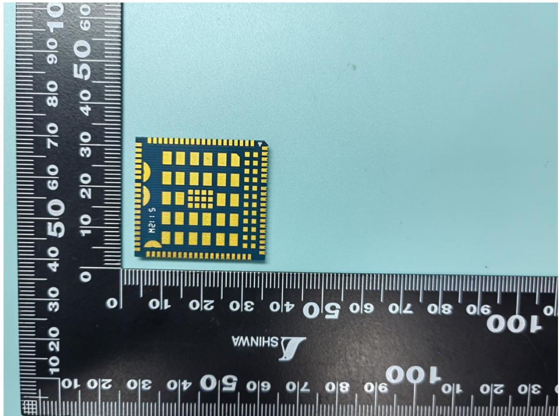
EC21-A_Bottom
