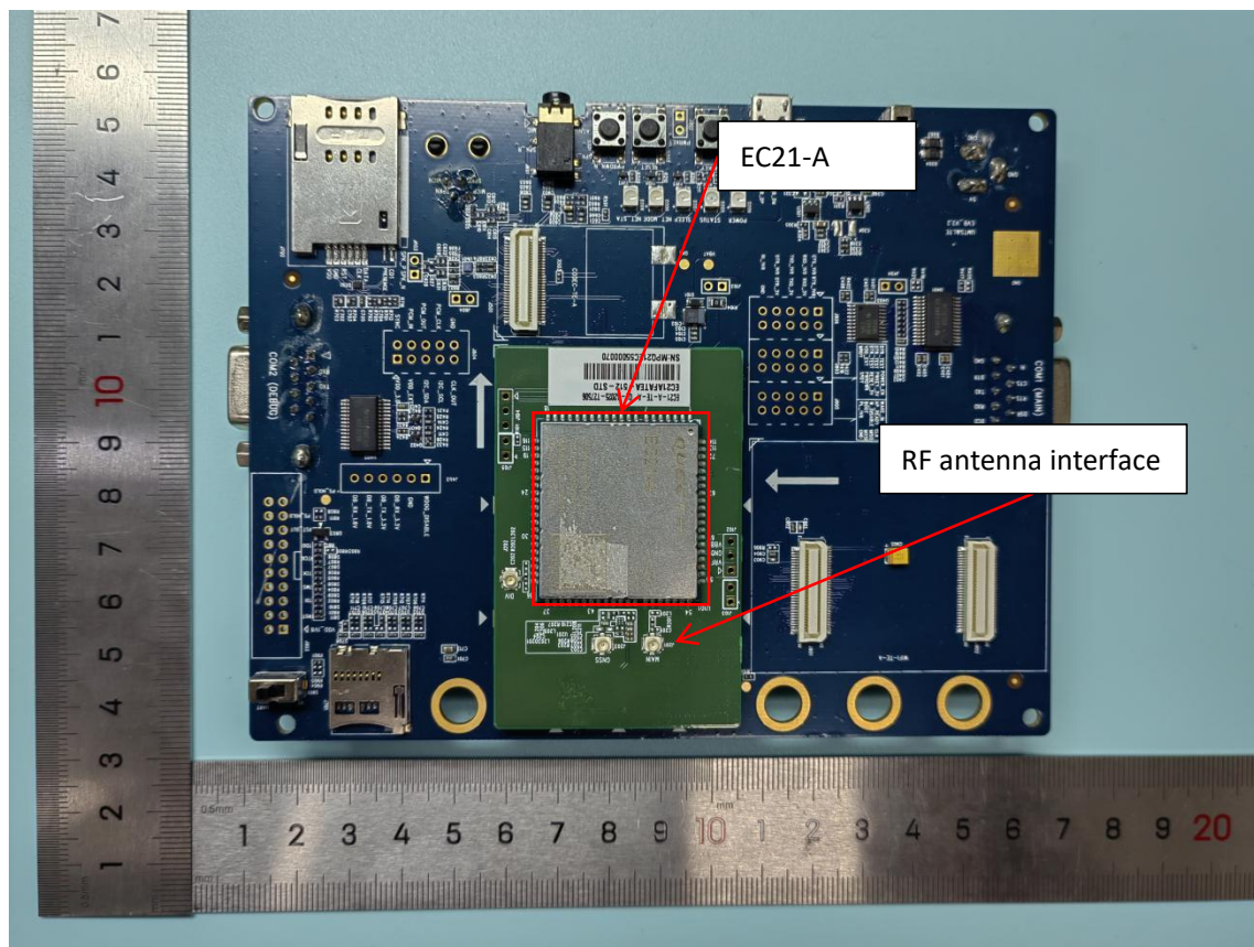
EC21-A + EVB_Top
