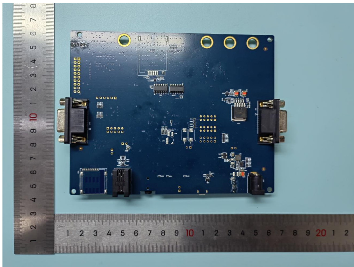
EC21-A + EVB_Bottom
