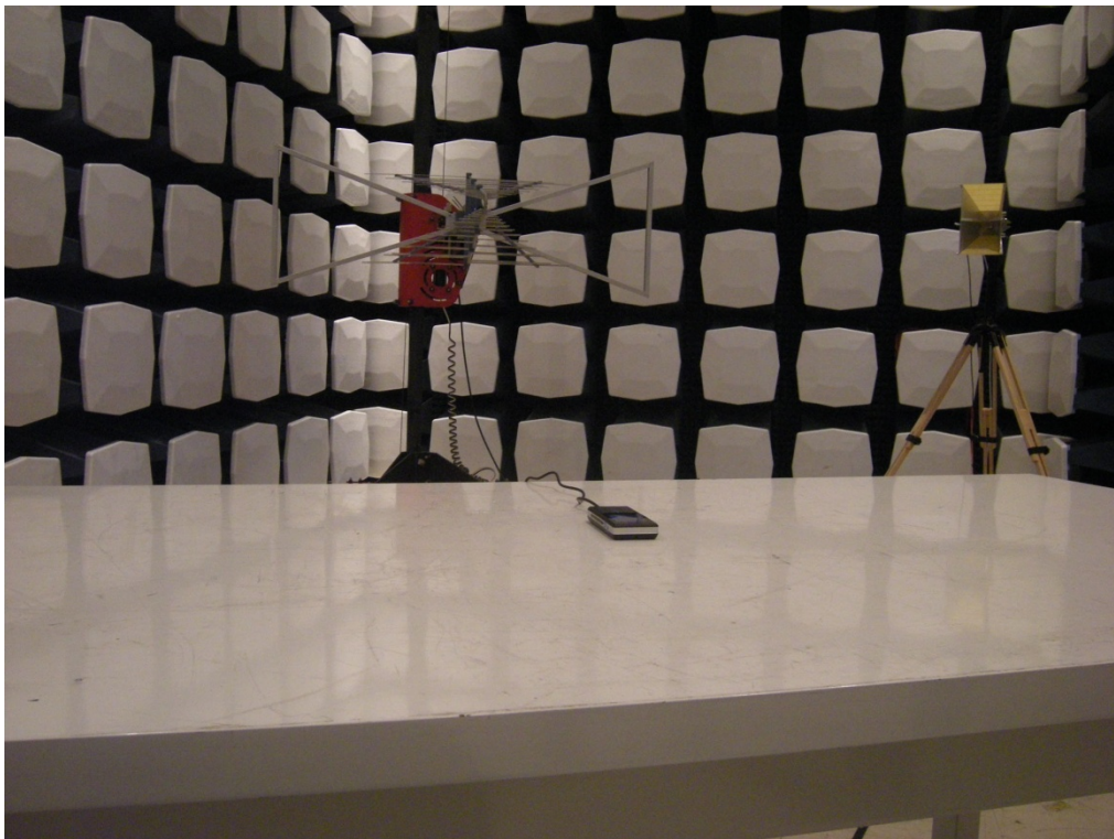
CE TEST
