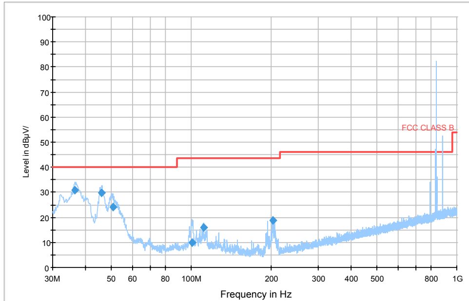
(Plot A: Test Antenna Vertical)
