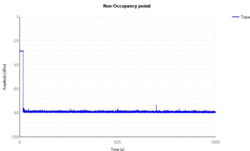
11ac 80MHz Mode 5690MHz
