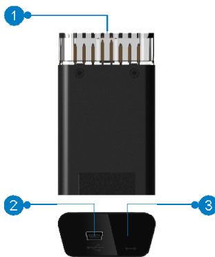
Fig. 1-2 VCI module
