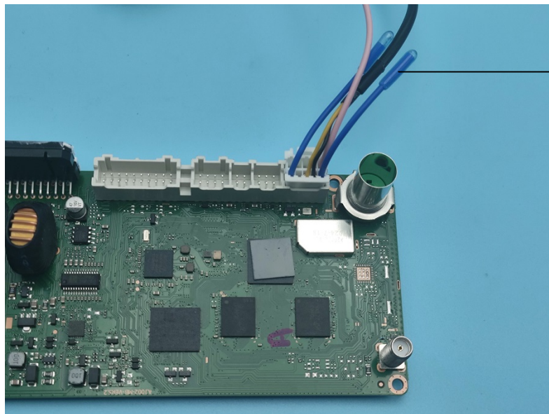
BT/WiFi antenna
