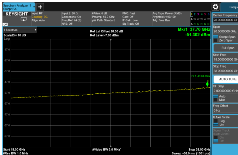
Channel: TOP, Modulation: QPSK, BW=15MHz, Range: 18GHz - 38GHz
