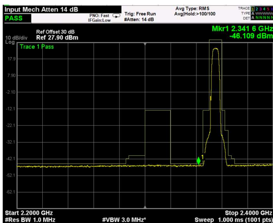
AWGN SIGNAL, 2.2GHz-2.4GHz
