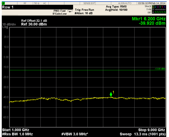
1GHz-9GHz
