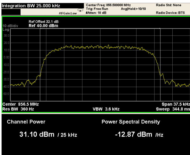
Mod. iDEN
