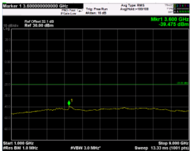
1GHz-9GHz
