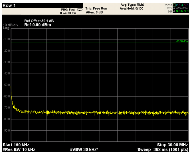
150kHz-30MHz
