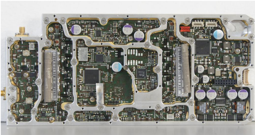
Up-link module
