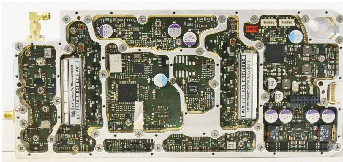
Up-link module
