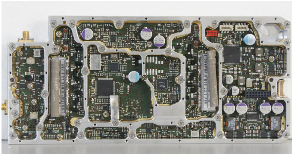
Up-link module
