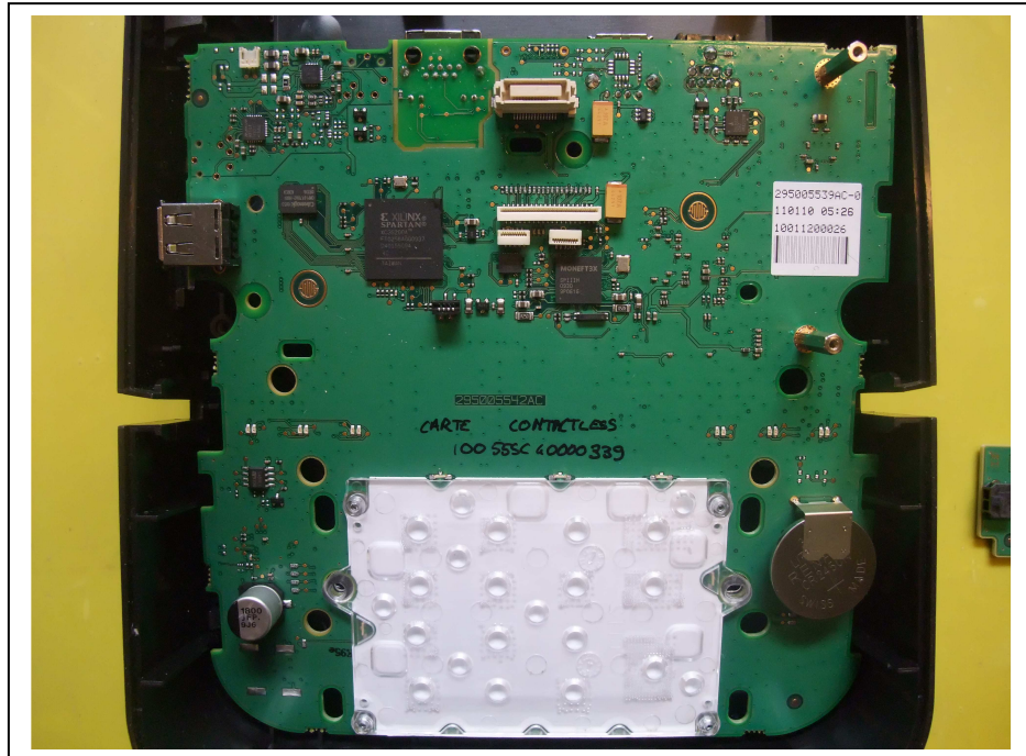
ISC 350 Mainbord 1
