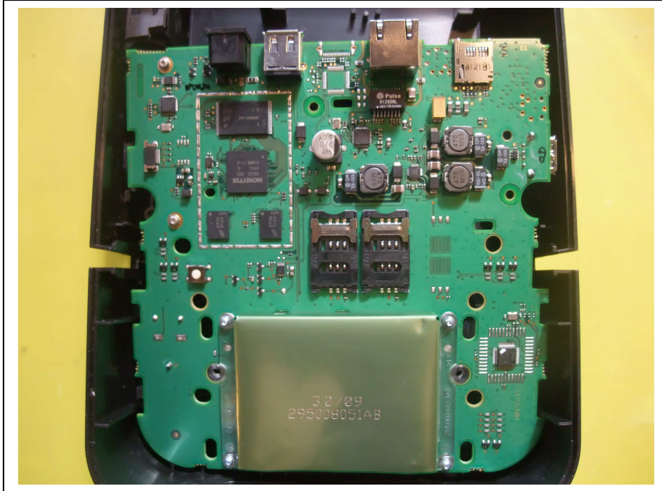
ISC 350 Mainbord 2
