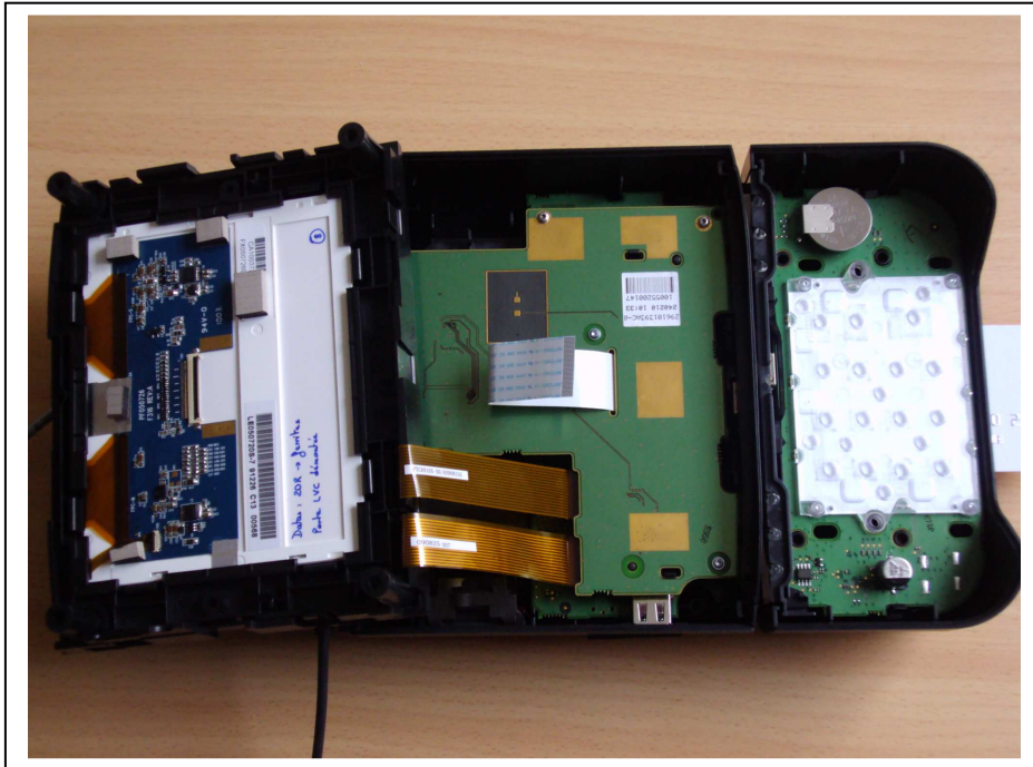
ISC 350 Overview
