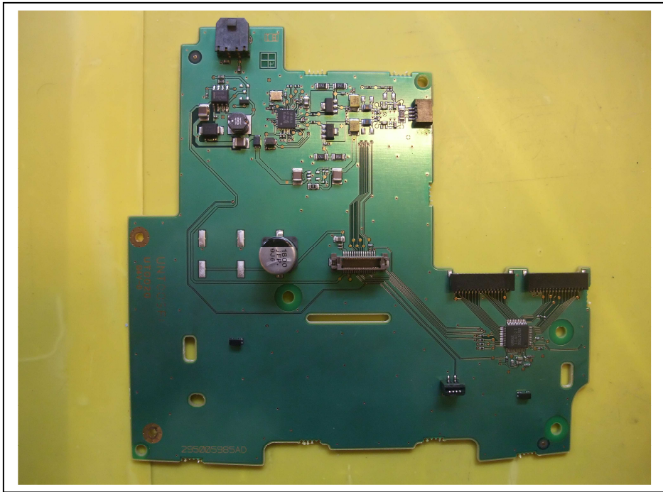
ISC 350 Topboard 1
