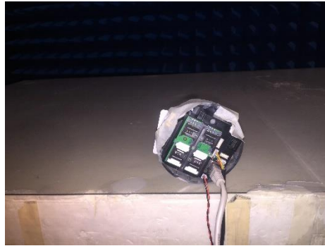
AXIS Z
