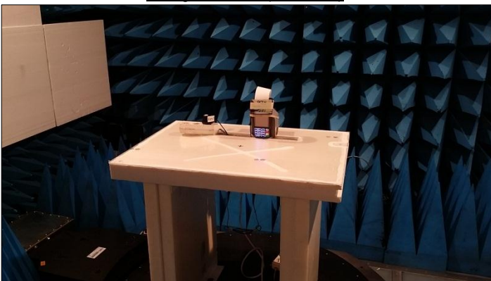
Configuration n°3 (Position Z)
