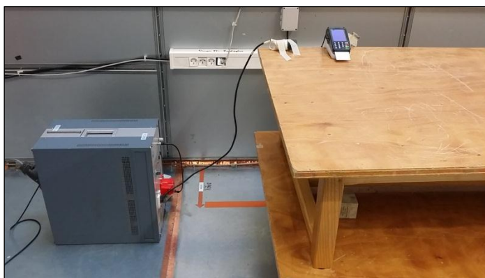
Configuration n°3 Test Setup
