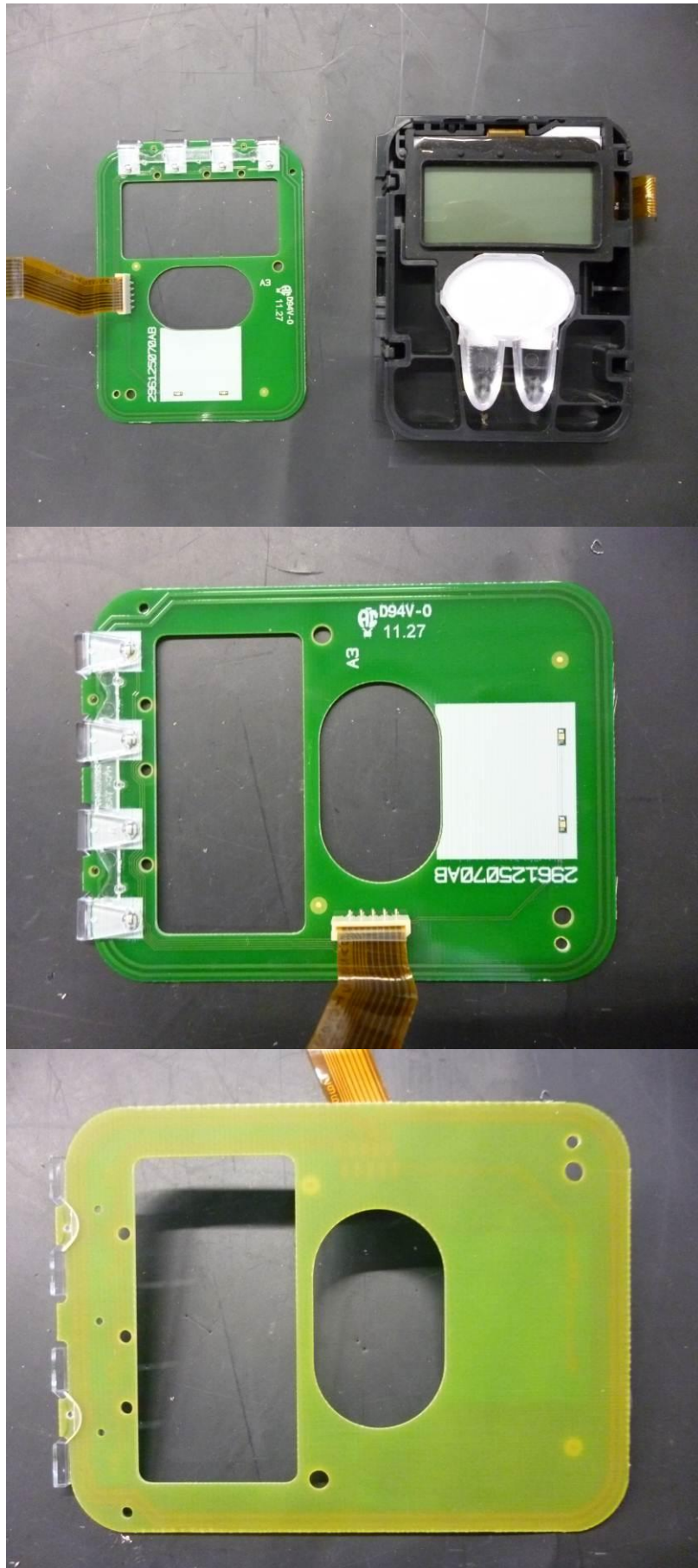
RFID antenna
