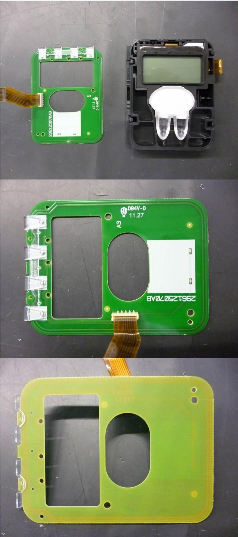
RFID antenna
