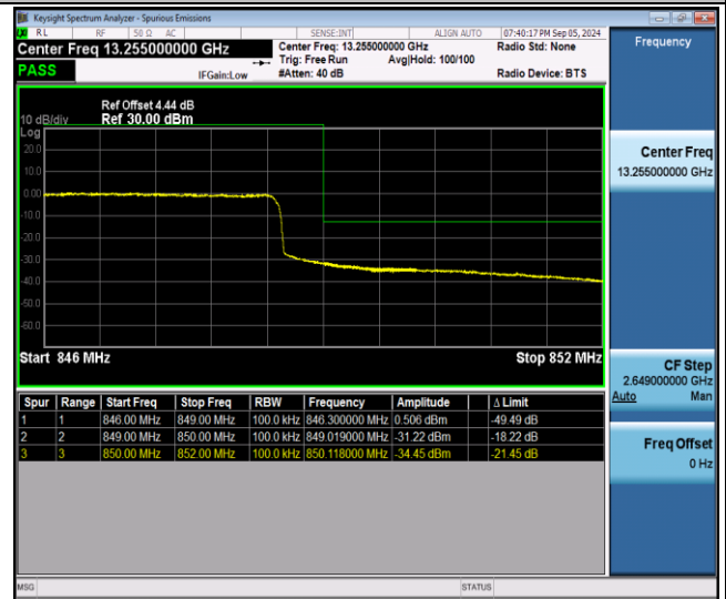
Band26(824-849)-10MHz-QPSK-26990-50RB#0-PASS
