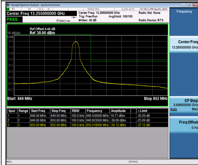
Band26(824-849)-10MHz-QPSK-26990-1RB#49-PASS
