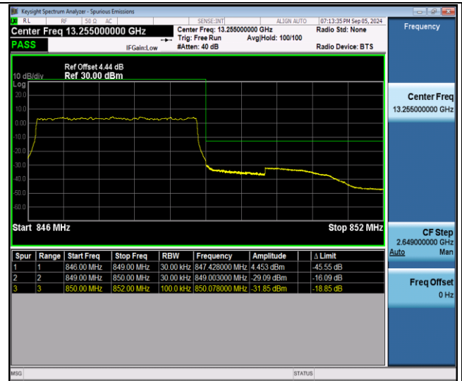
Band26(824-849)-3MHz-QPSK-27025-15RB#0-PASS
