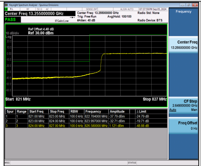
Band26(824-849)-10MHz-QPSK-26840-50RB#0-PASS
