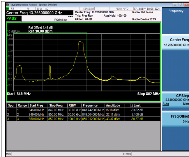
Band26(824-849)-3MHz-QPSK-27025-1RB#14-PASS
