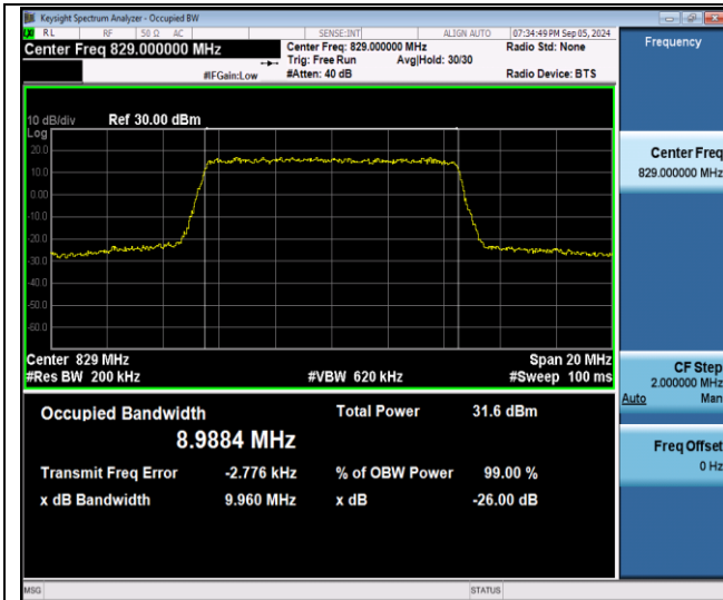
Band26(824-849)-10MHz-QPSK-26840-50RB#0-PASS
