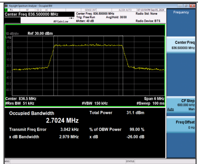
Band26(824-849)-3MHz-QPSK-26915-15RB#0-PASS
