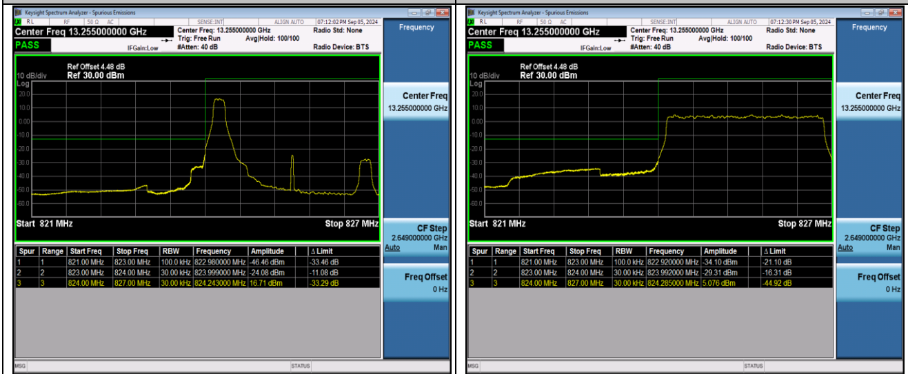
Band26(824-849)-3MHz-QPSK-26805-1RB#0-PASS
