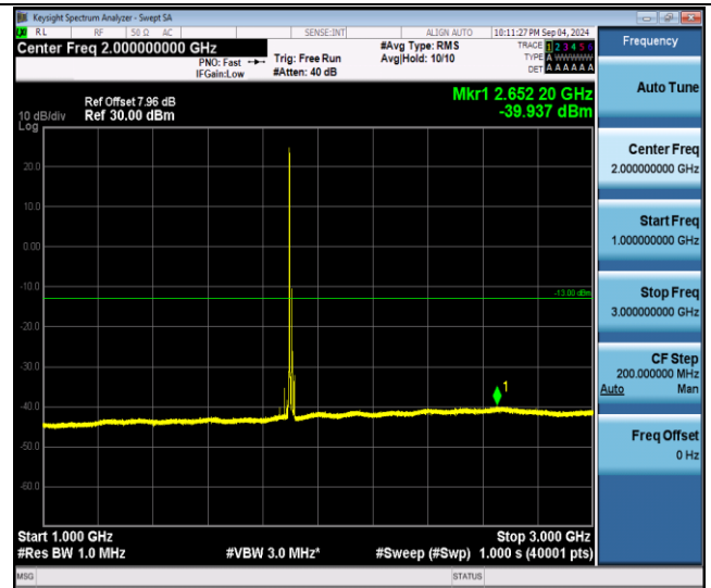
Band25-20MHz-QPSK-26590-1RB#0-1000~3000-PASS
