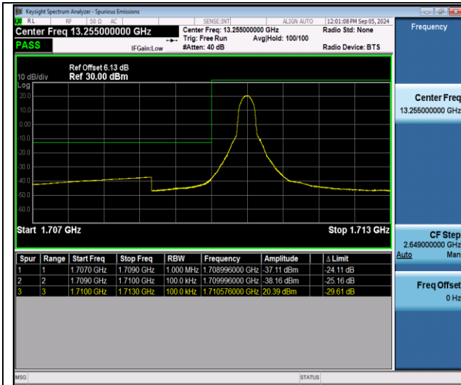
Band4-10MHz-QPSK-20000-1RB#0-PASS
