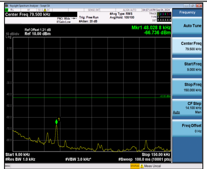
GPRS1900-661-0-0.009~0.15MHz-PASS
