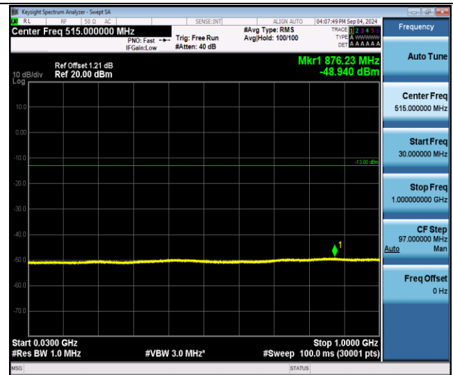
GPRS1900-661-0-30~1000MHz-PASS
