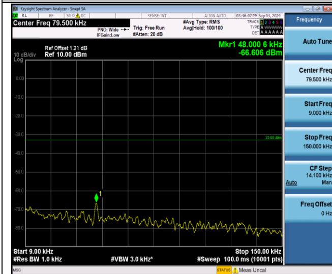
EGPRS850-251-8-0.009~0.15MHz-PASS
