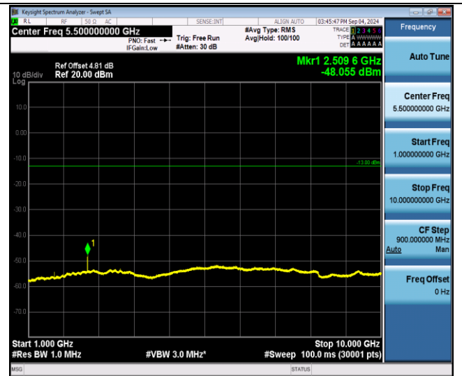
EGPRS850-190-8-1000~10000MHz-PASS
