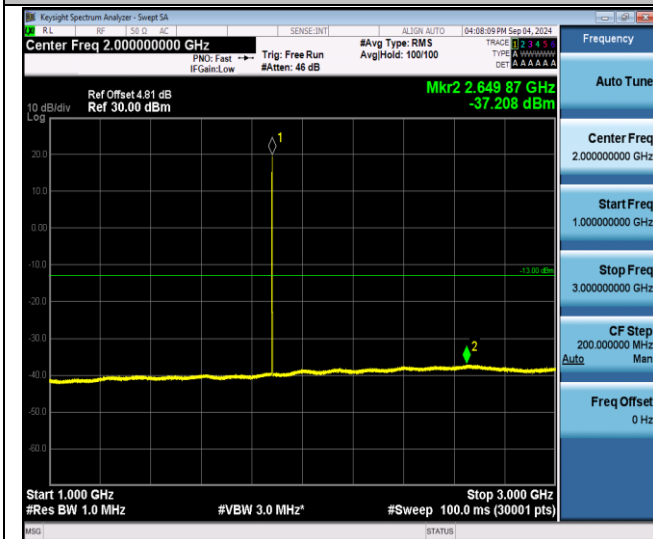
GPRS1900-661-0-1000~3000MHz-PASS
