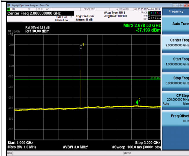
EGPRS1900-810-2-1000~3000MHz-PASS
