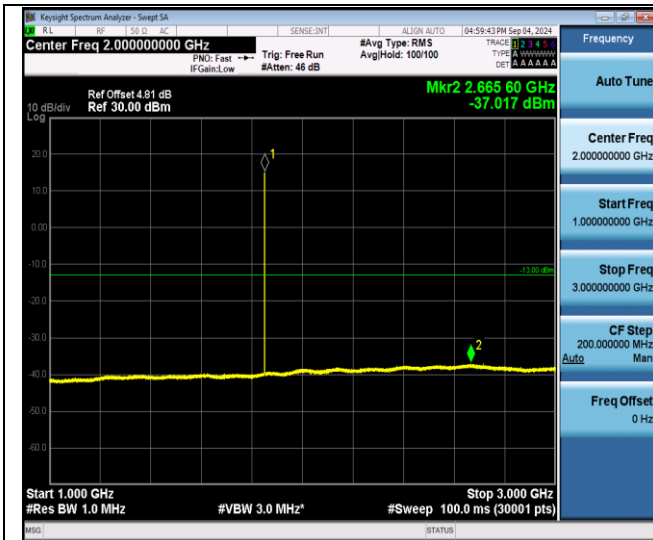
EGPRS1900-512-2-1000~3000MHz-PASS
