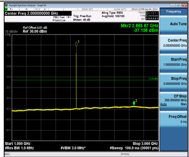
EGPRS1900-661-2-1000~3000MHz-PASS
