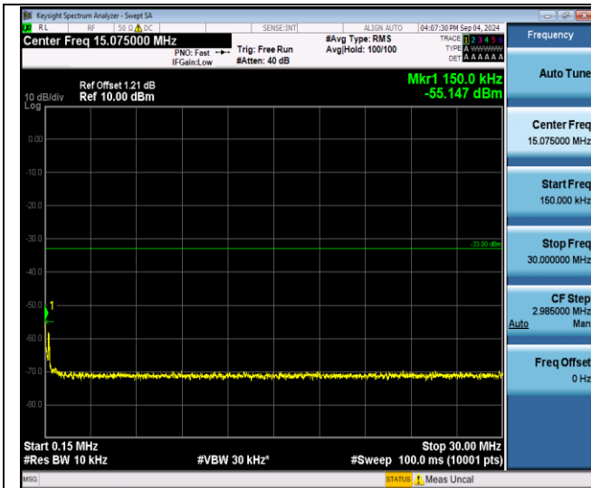
GPRS1900-661-0-0.15~30MHz-PASS
