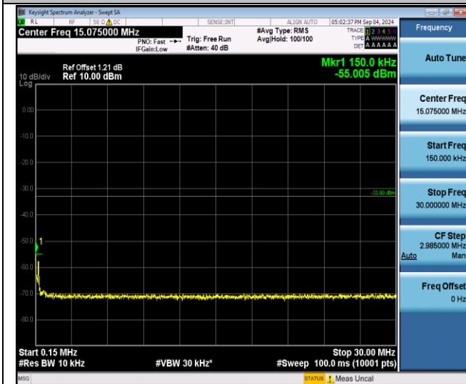
EGPRS1900-810-2-0.15~30MHz-PASS
