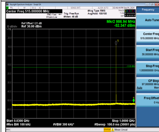
EGPRS850-251-8-30~1000MHz-PASS
