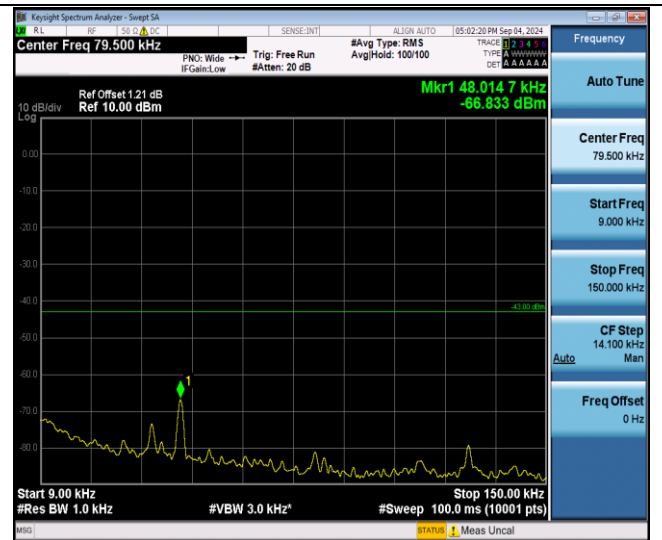
EGPRS1900-810-2-0.009~0.15MHz-PASS
