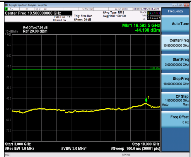
GPRS1900-661-0-3000~18000MHz-PASS
