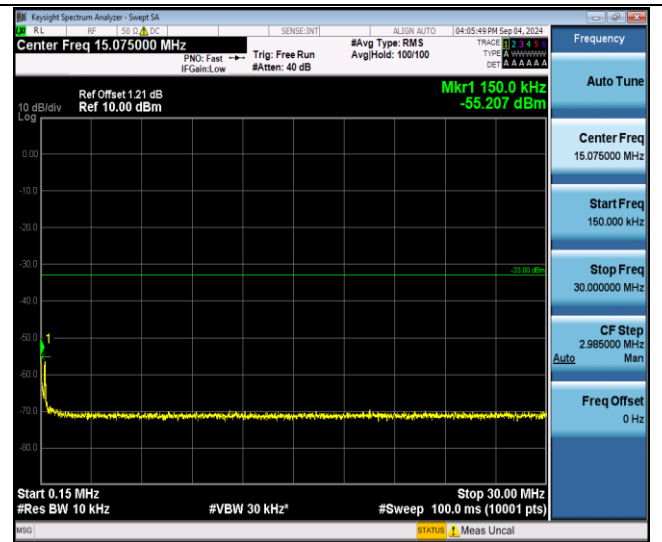
GPRS1900-512-0-0.15~30MHz-PASS
