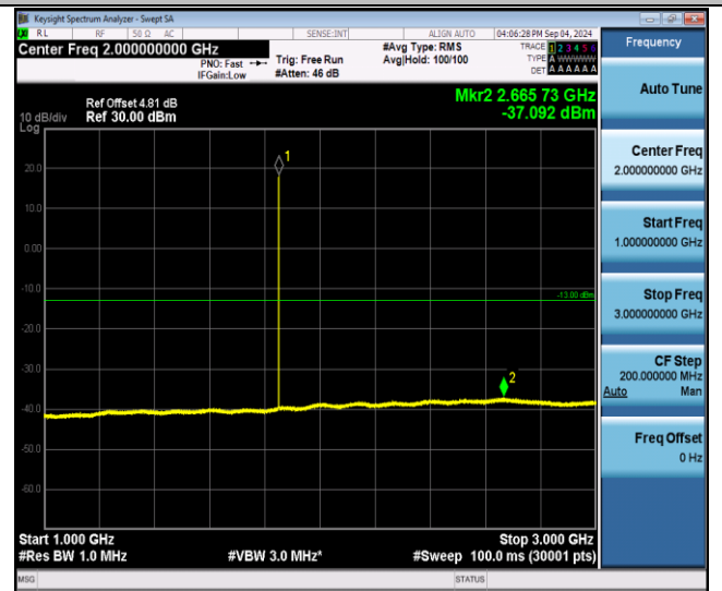
GPRS1900-512-0-1000~3000MHz-PASS
