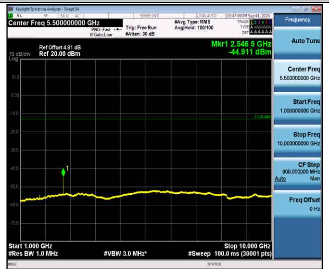
EGPRS850-251-8-1000~10000MHz-PASS
