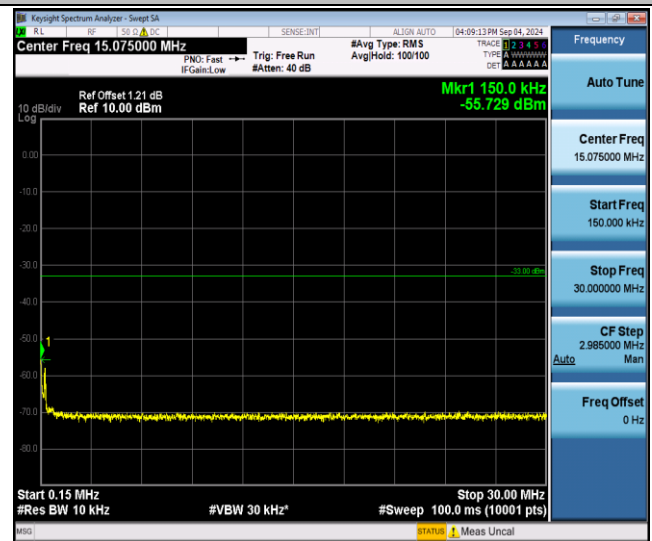
GPRS1900-810-0-0.15~30MHz-PASS
