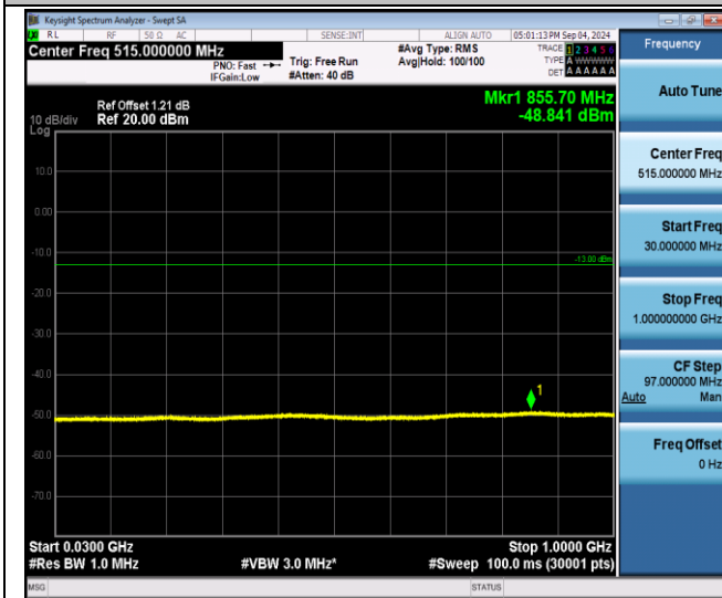
EGPRS1900-661-2-30~1000MHz-PASS
